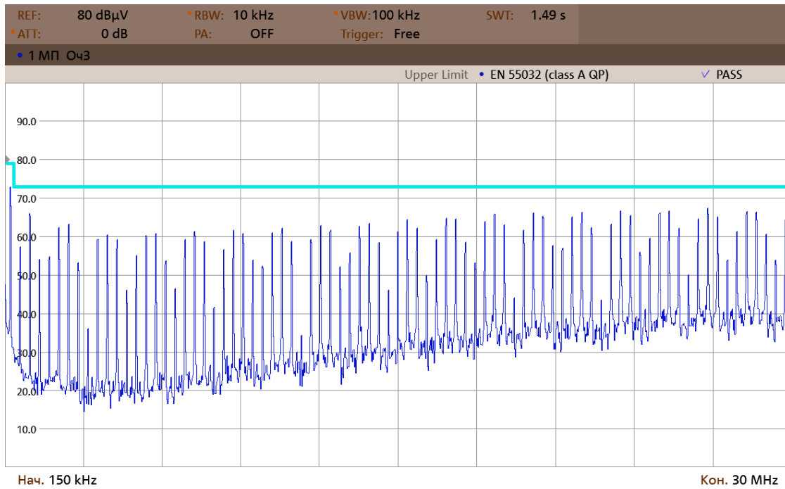
Рис. 50. Спектрограмма соответствия EN55032 Class A (0,15–30 МГц).
