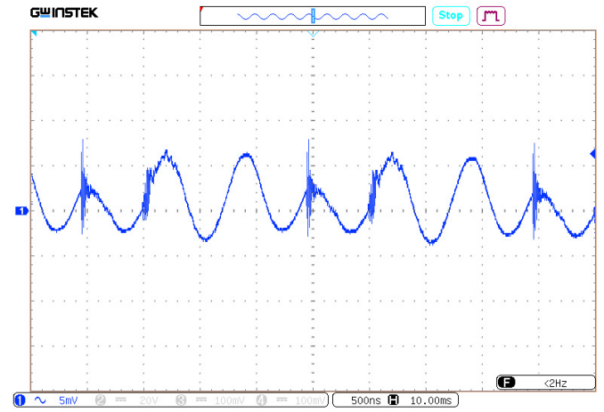
Рис. 43. Пульсации U_{\text{ВЫХ.НОМ}} .
