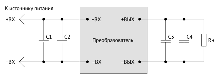
Рис. 2. Схема включения VDR15, VDR25.
