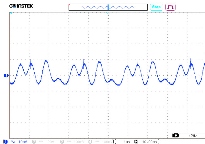
Рис. 35. Пульсации U_{\text{ВЫХ.НОМ}} .
