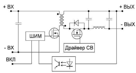
Рис. 1. Топология VDR15, VDR25.
