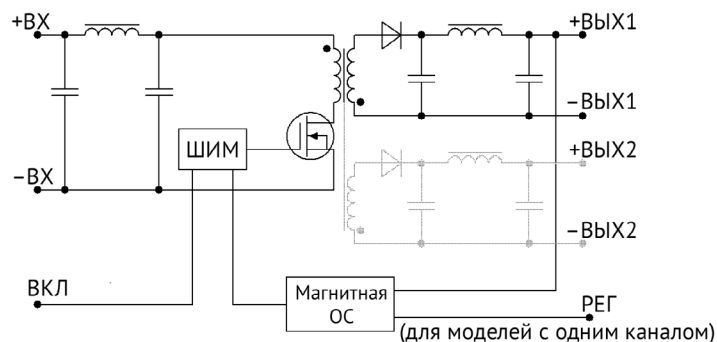
Рис. 1. Топология VDV12.
