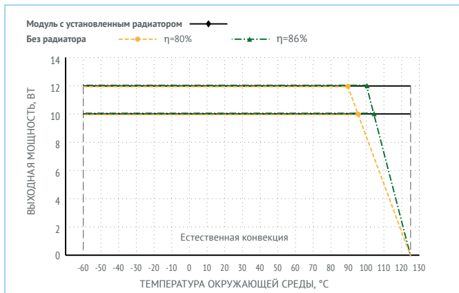
Рис. 7. Тепловая кривая VDV12.
