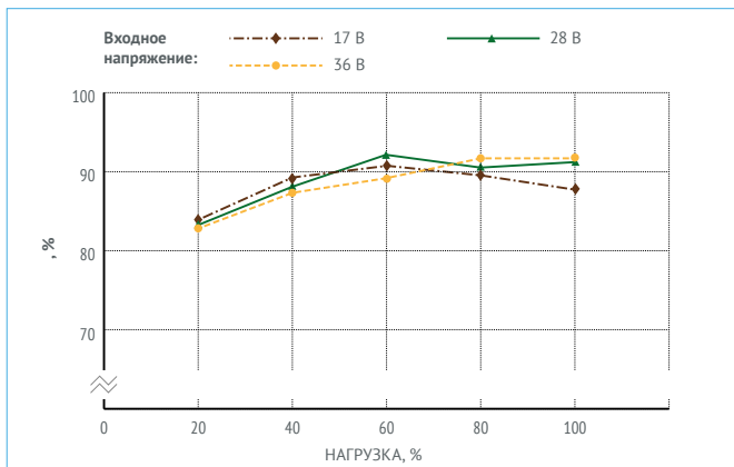
Рис. 6 (а). КПД VDV80-1V28.
