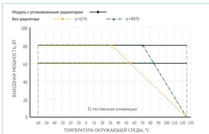
Рис. 7. Тепловая кривая VDV80.
