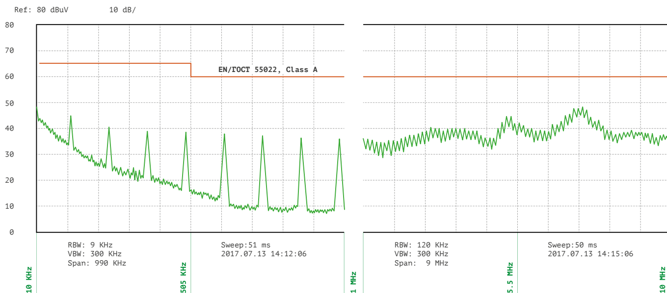
Рис. 8. Спектрограмма радиопомех VDV80-1V05 с типовой схемой подключения.
