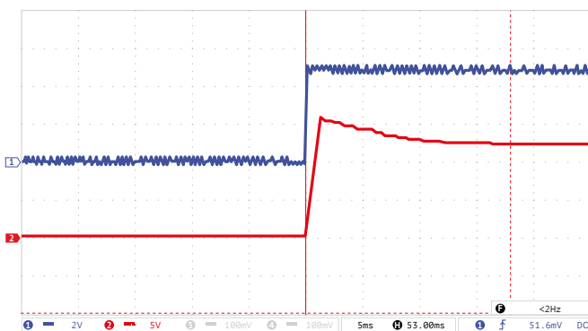
Рис. 9 (а). Осциллограмма установления выходного напряжения с момента подачи команды дистанционного управления.
