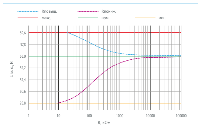
Рис. 10. График зависимости для VDRW100N36.
