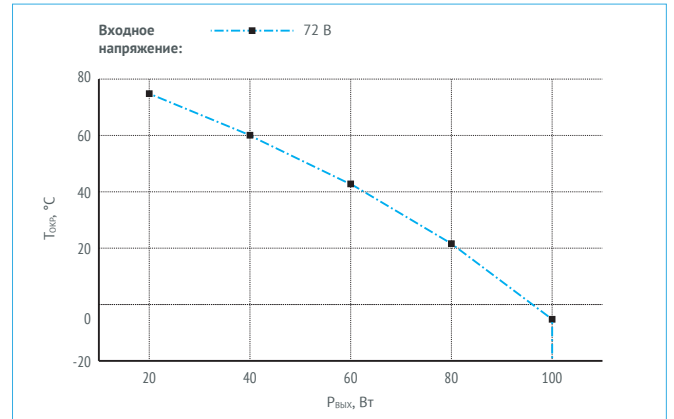
Рис. 13. Зависимость снижения P_{\text{ВЫХ}} от T_{\text{ОКР}} .
