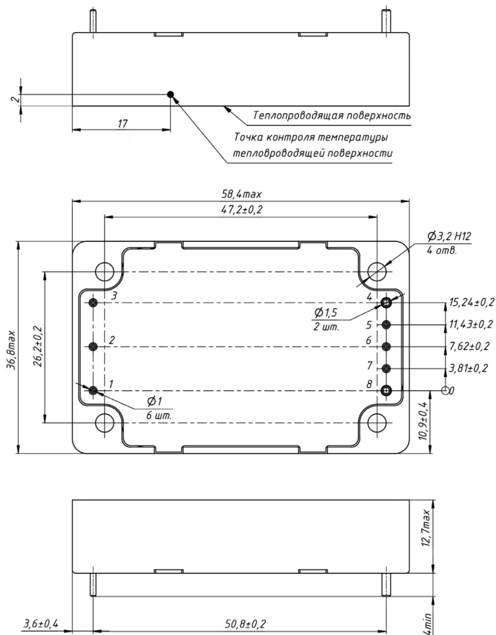
Рис. 30. Исполнение 1/4 Brick.
