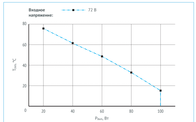
Рис. 15. Зависимость снижения P_{\text{ВЫХ}} от T_{\text{ОКР}} .
