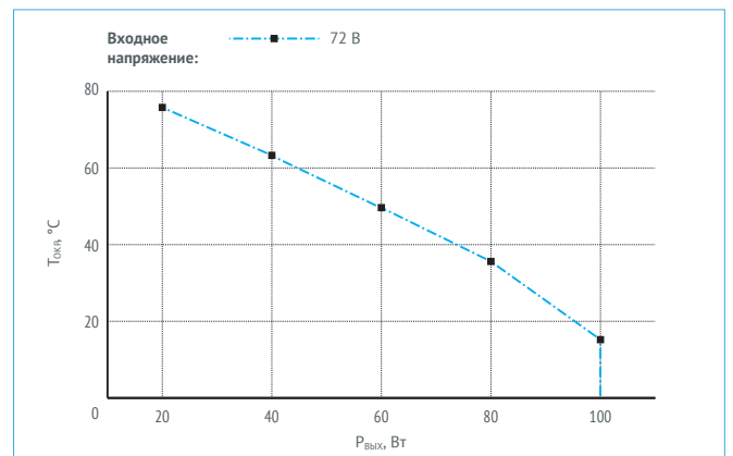
Рис. 17. Зависимость снижения P_{\text{ВЫХ}} от T_{\text{ОКР}} .
