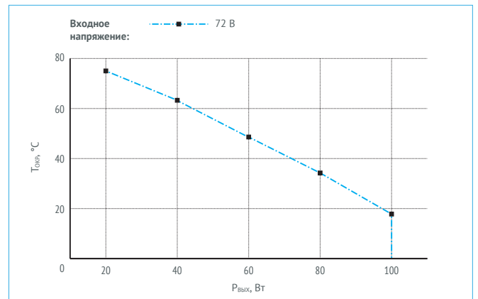
Рис. 19. Зависимость снижения P ВЫХ от T ОКР .
