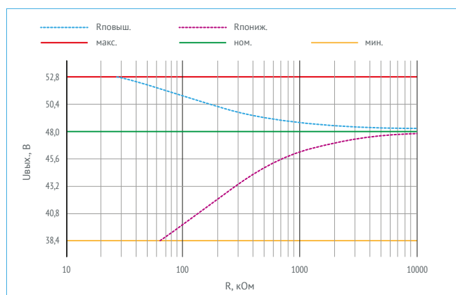
Рис. 11. График зависимости для VDRW100N48.
