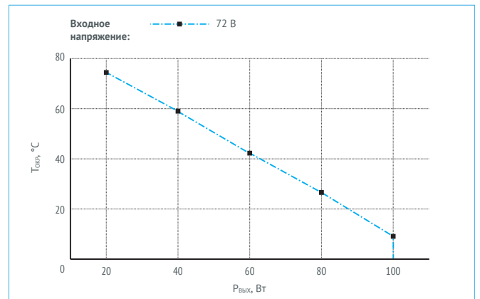
Рис. 21. Зависимость снижения P ВЫХ от T ОКР .
