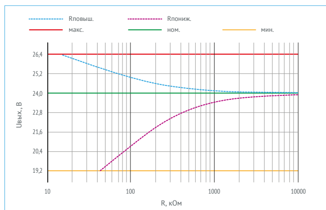
Рис. 9. График зависимости для VDRW100N24.
