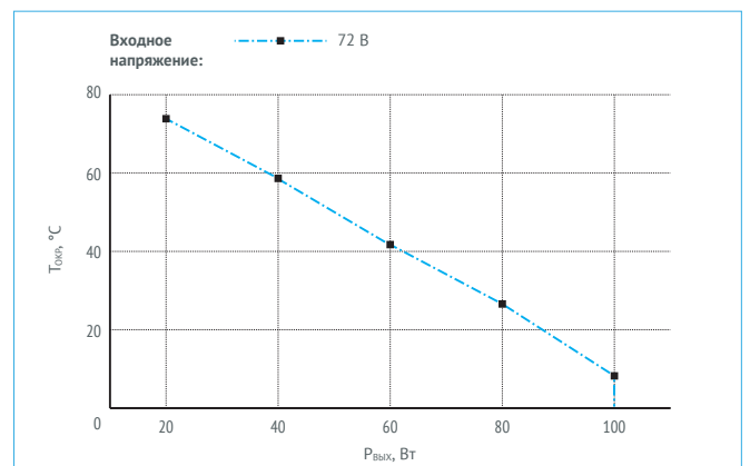
Рис. 23. Зависимость снижения P ВЫХ от T ОКР .
