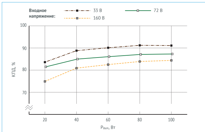
Рис. 20. КПД.
